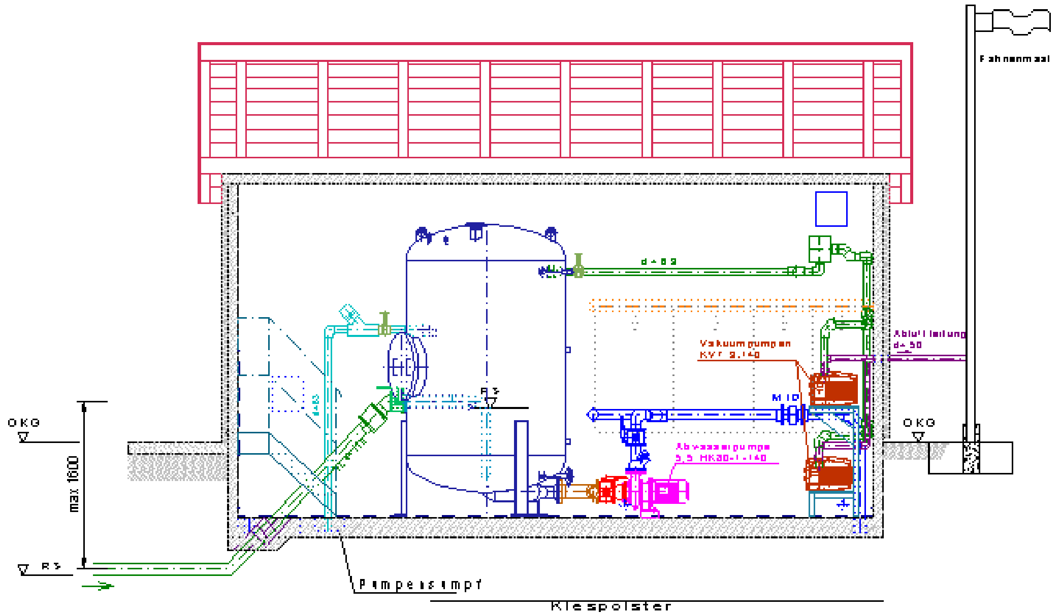
Schnitt A-A (Technologie)
