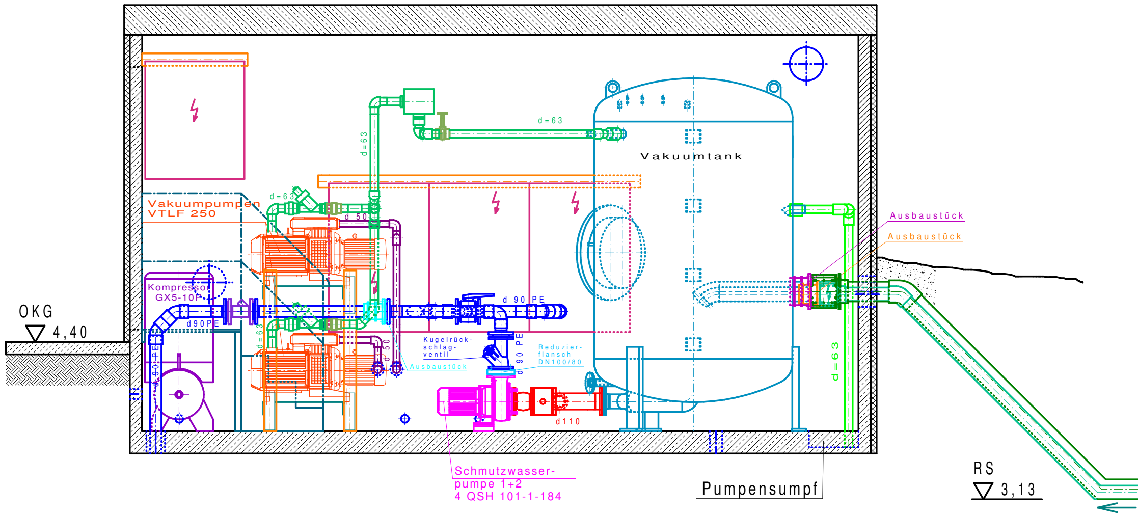
Schnitt A-A (Technologie)
